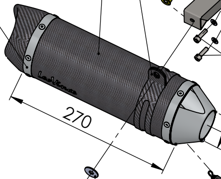
2x Allen screw M8X20 T.C.Z.B. Cod.200722
