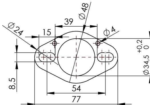
S.s. Flange Cod.206443R
