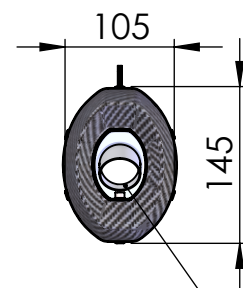
Db-killer N°52B Cod.308437801R
