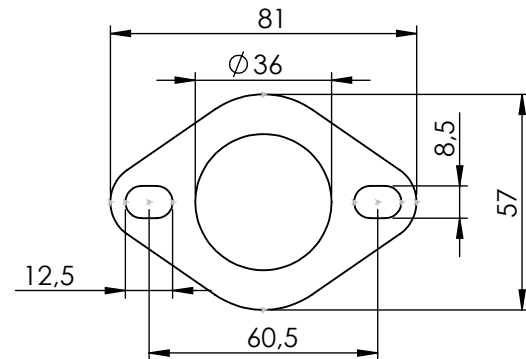
S.S. Flange P/N 201299
