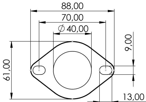
S.S. Flange 38C P/N 207104
