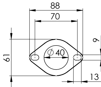
S.S. Flange 38C P/N 207104
