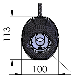
dB-Killer n°62 kit P/N 3014259801R
