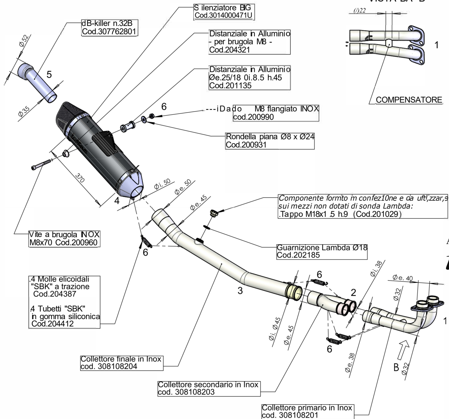
VISTA DA "B"
