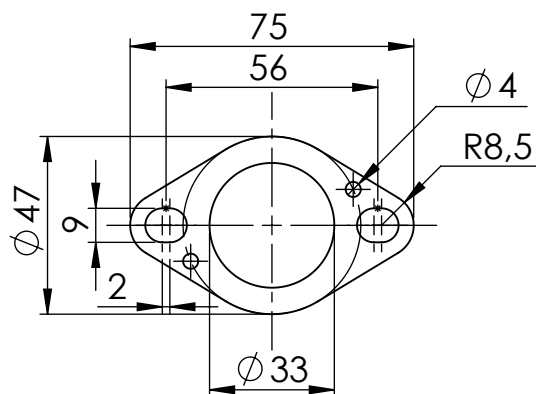
Flange 45E Cod.205267
