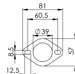
S.S. Flange 25B P/N 200560
