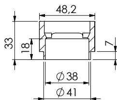
S.s.bushing
