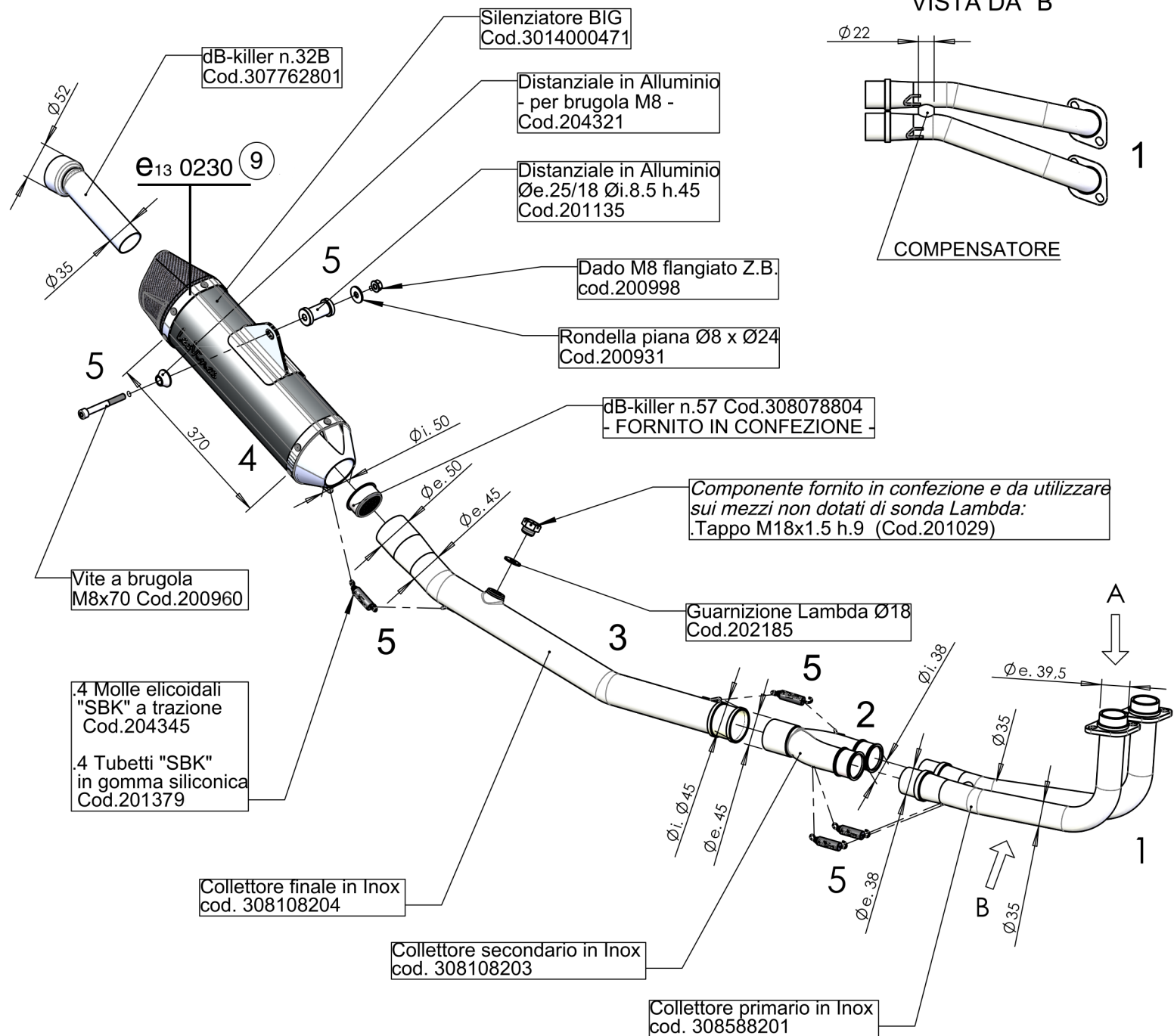
VISTA DA "B"
