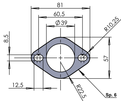
VISTA DA "A" Flange "25B"
