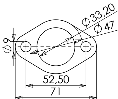
S.s. Flange "43A" Cod.201208
